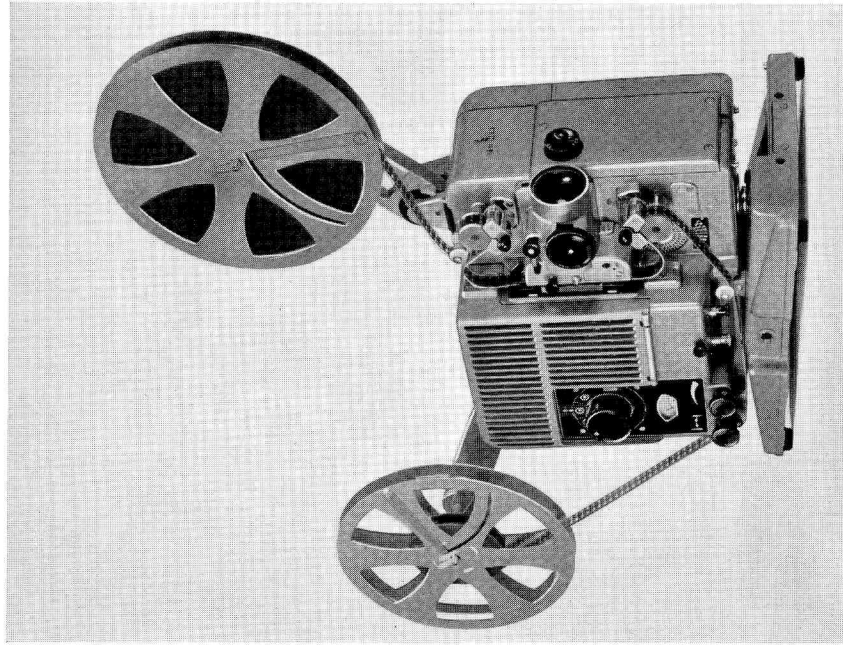
Bild 1 Ansicht der Bedienungsseite
